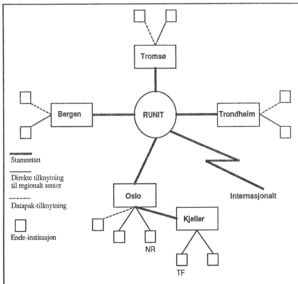
Figur 3: Stamnettet i UNINETT
